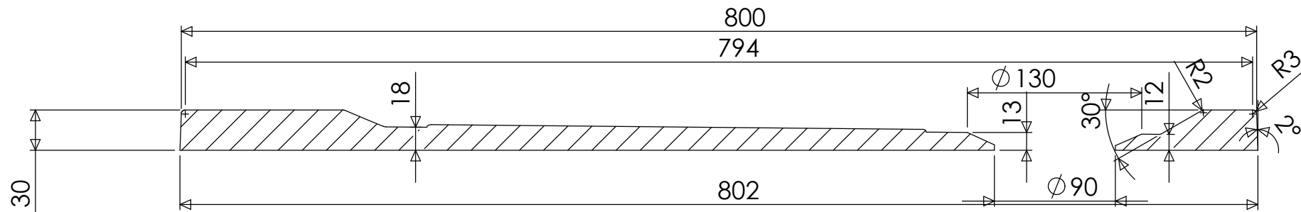
SECTION B-B SCALE 1 : 4
