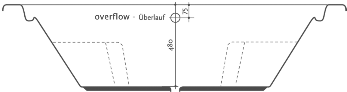
Tiefschnitt - vertical section
